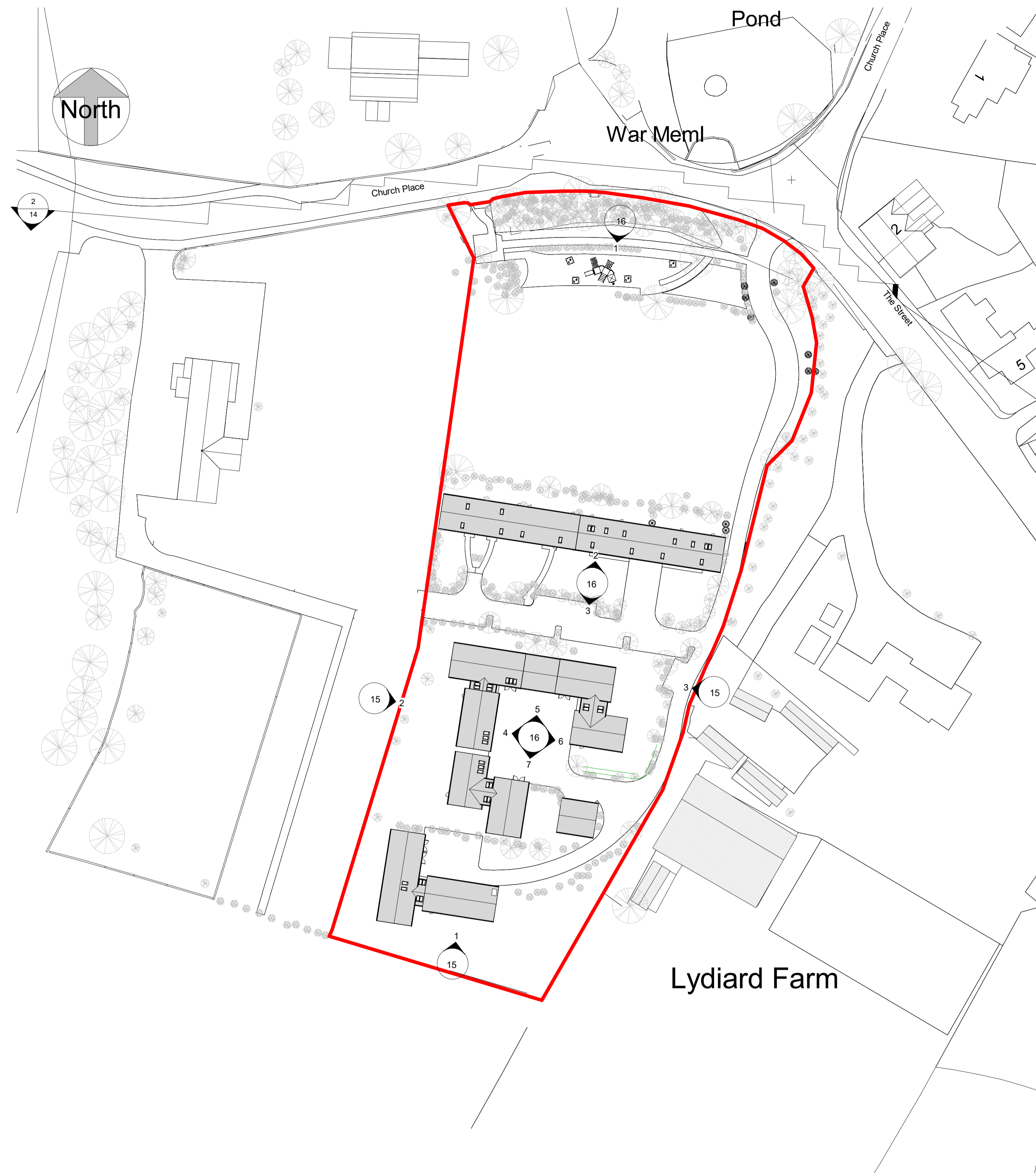
2 Block Plan 1 : 500
